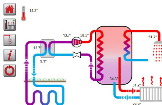
Eksempel for jordvarme
